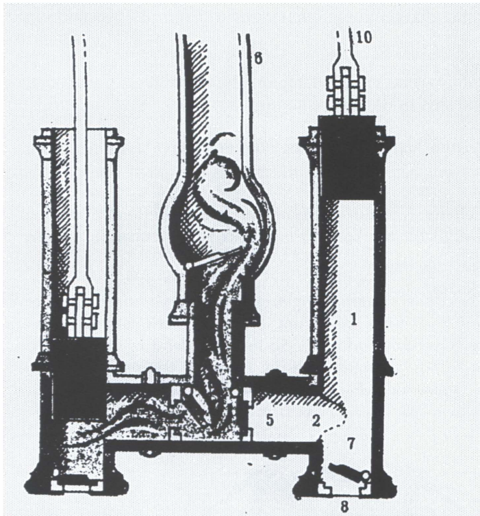
Schematische Darstellung eines anderen Heron-Projekts, wie es sich die Wissenschaftler vorstellen: Feuerspritzen-Druckpumpe aus Bronze. (1) Zylinder (2) Verbindungsstück (3) Verbindungstunnel zum Windkessel (4) Windkessel (5) Druckventile (6)
