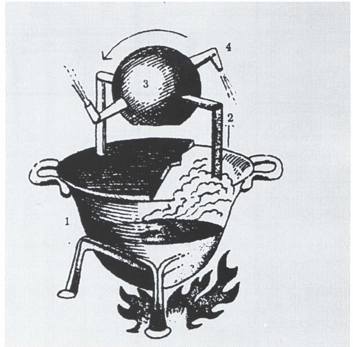
Die Aeolopile des Heron
